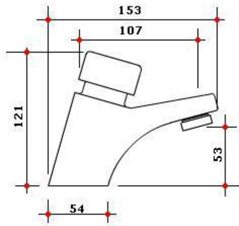
Torneira c/ fechamento automático Dimensões em milímetros
