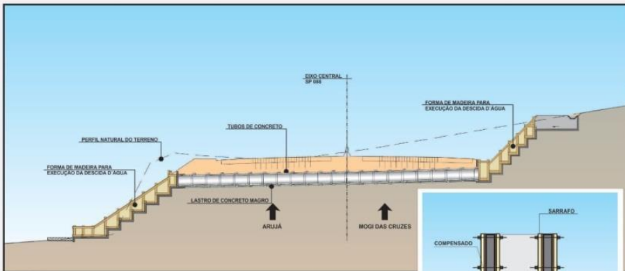
CORTE - EXECUÇÃO DA DESCIDA D'ÁGUA EM DEGRAUS
