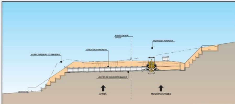
CORTE - ASSENTAMENTO DE TUBOS DE CONCRETO (BSTC)
