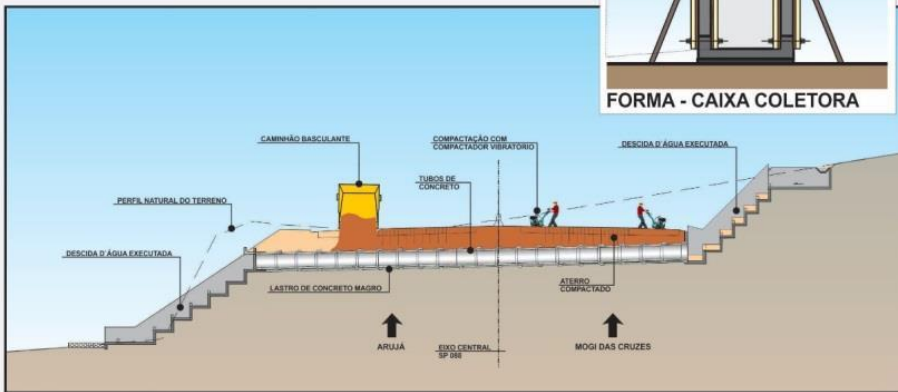
CORTE - REATERRO E COMPACTAÇÃO DA VALA
