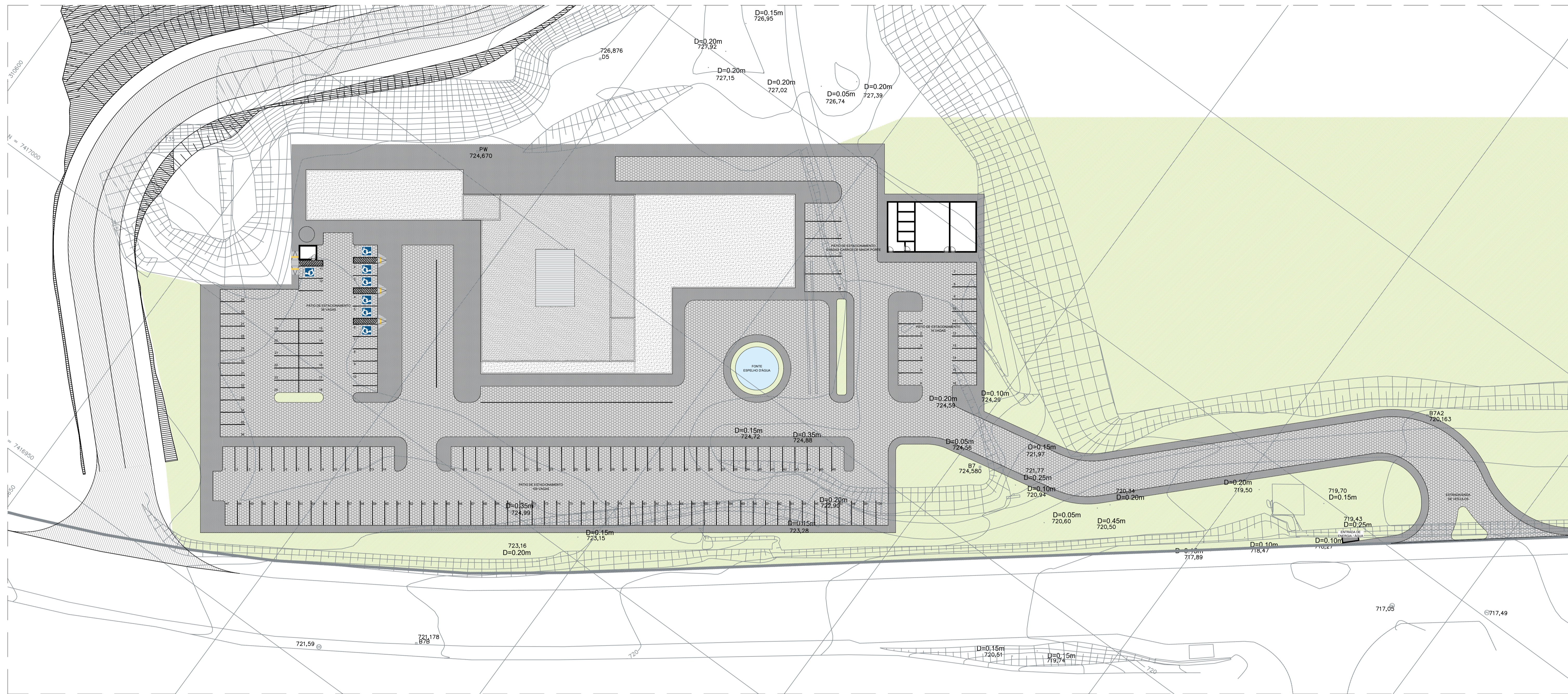
1 PLANTA DE IMPLANTAÇÃO GERAL | LOCALIZAÇÃO Escala 1:400
